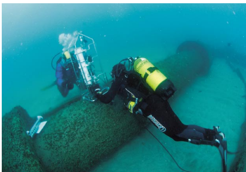
Figura 66. Medición de parámetros en tramo difusor del emisario de salmueras de la desaladora de Blanes (Girona) mediante CTD. Por cortesía de Ecoproges S.L. Fotografos: Joan Carles Fluxà y Jordi Chías
