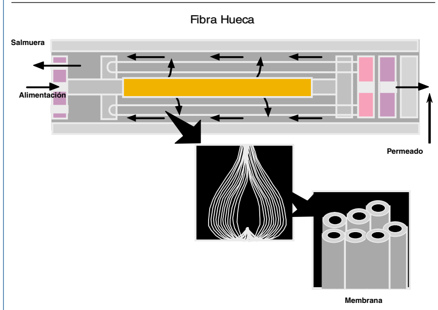
Figura 19. Esquema de la configuración fibra hueca
