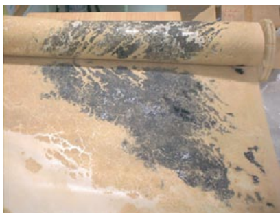
Figura 55. Depósitos de materia orgánica y biopelícula en la superficie de la membrana
