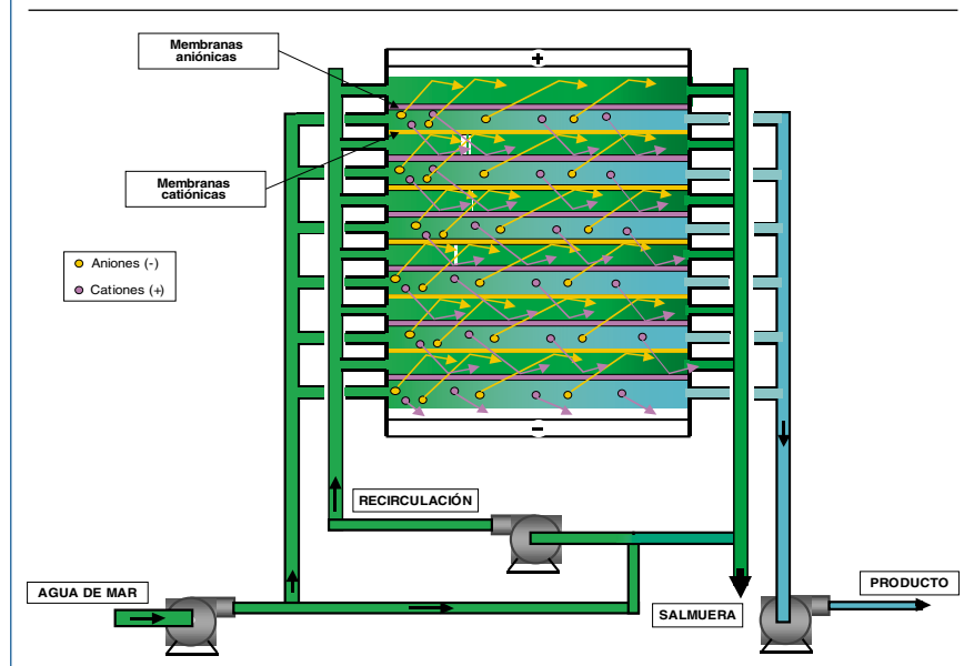
Figura 35. Diagrama del funcionamiento de la electrodiálisis reversible. Por cortesía de ECOAGUA INGENIEROS
