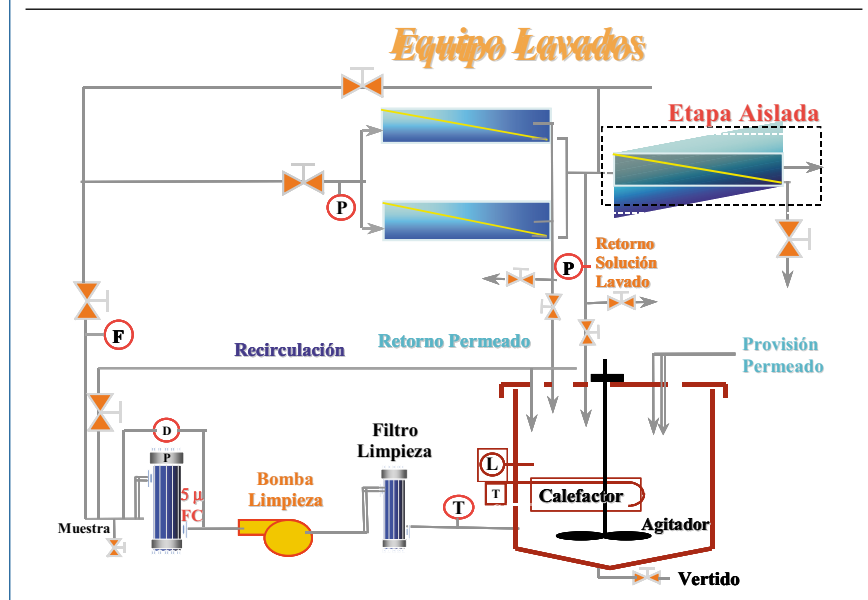
Figura 57. Esquema general de limpieza química de una instalación de membranas
