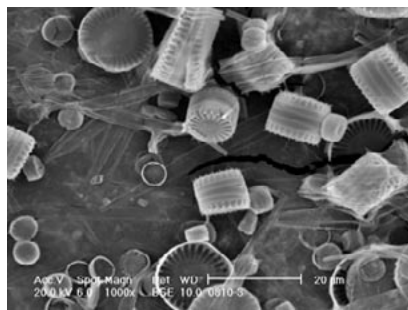
Figura 56. Microfotografía SEM de la superficie de una membrana de ósmosis inversa. Presencia de diatomeas y otros microorganismos
