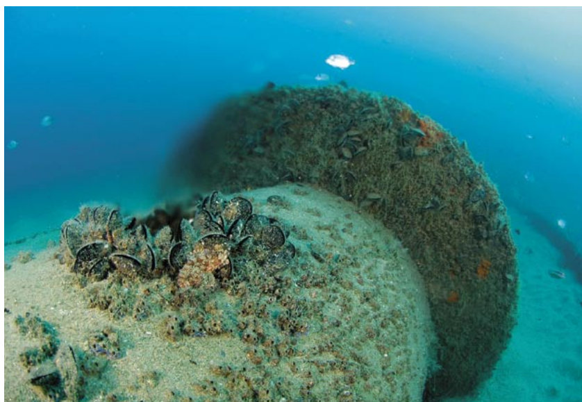
Figura 65. Tramo difusor del emisario de salmueras de la desaladora de Blanes (Girona). Por cortesía de Ecoproges S.L. Fotografos: Joan Carles Fluxà y Jordi Chías
