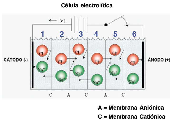
Figura 34. Pila de electrodiálisis. Por cortesía de GE Water & Process Technologies
