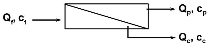
Figura 22. Esquema de balance de materia. El rectángulo expresa la planta en su conjunto
